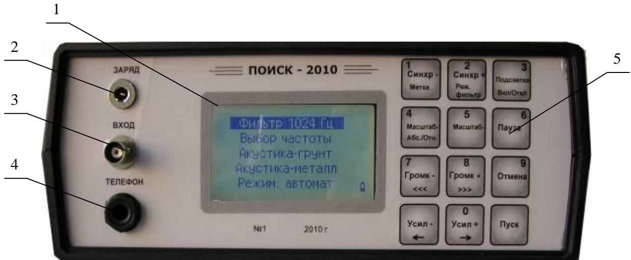
Рисунок 9. Приемник «ПОИСК-2006м». Панель лицевая.
